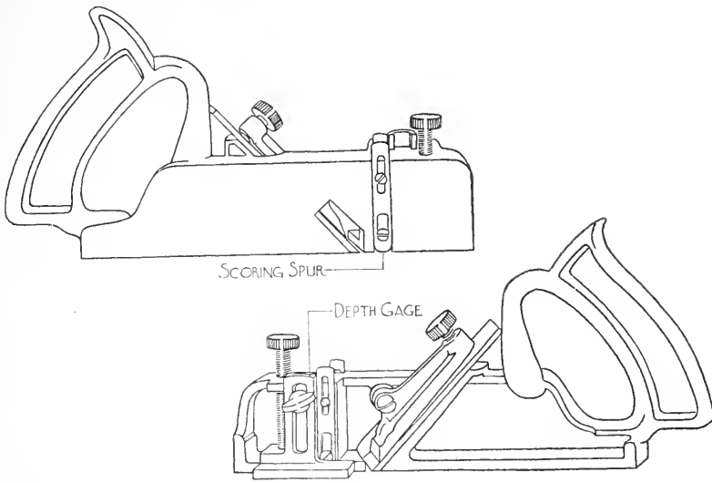
FIG. 70. DADO PLANE.
